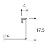
■ 製品図
