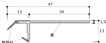
■ 製品図
