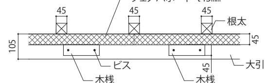
下から見たアングル固定位置のイメージ
