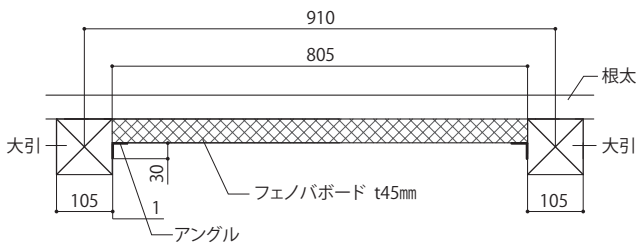
アングルを使用した場合
