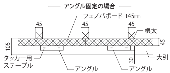
木棧固定の場合
