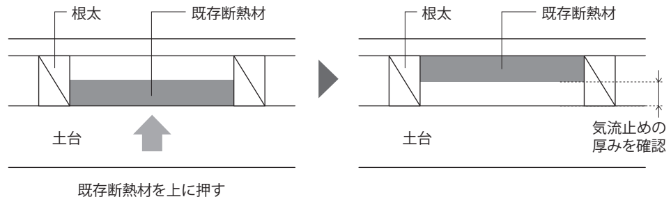
気流止めの施工
