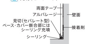
6 出隅
