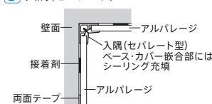
7 ジョイント
