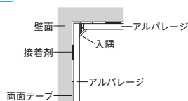
5 入隅
