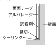
5 入隅
