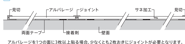
7 ジョイント
