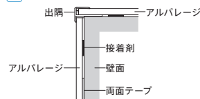
6 出隅
