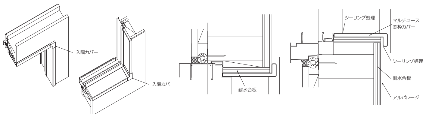
■縦枠－横枠(上枠)、横枠(下枠) 納まり
