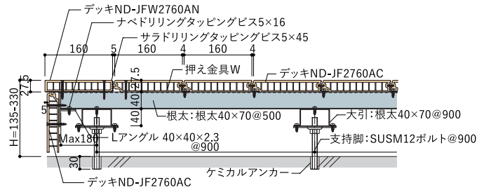
B-B断面図
