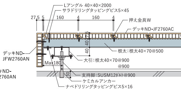
B-B断面図
