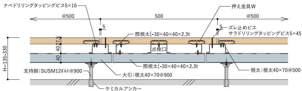
C-C断面図
