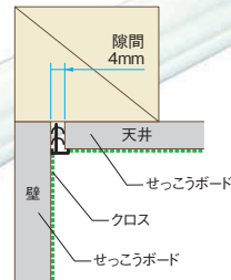
クロス後貼り施工
