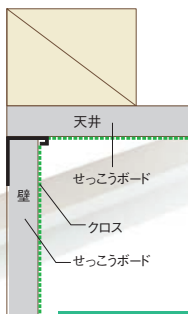
天井勝ち 納まり例
