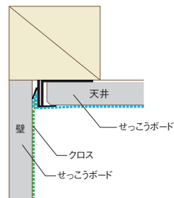
壁勝ち 納まり例
