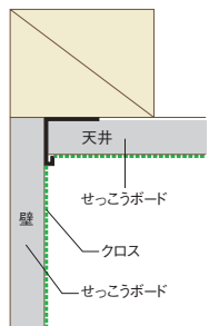
壁勝ち 納まり例
