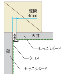
クロス先貼り施工
