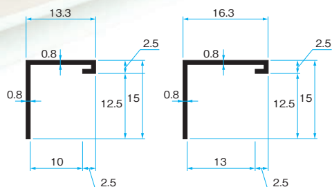
スツキリ見切 10
