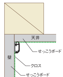
壁勝ち 納まり例
