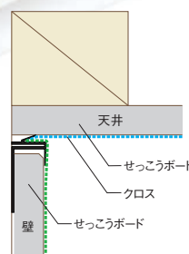
天井勝ち 納まり例
