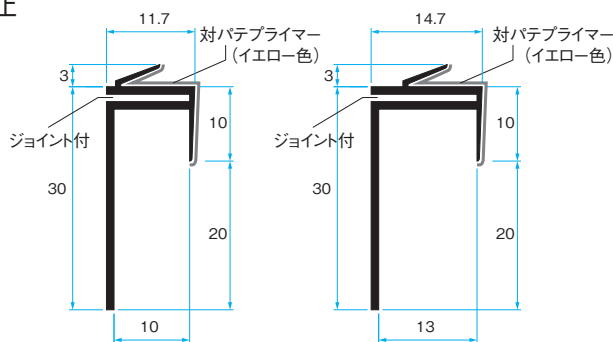
先付けクロスフリー見切 10
