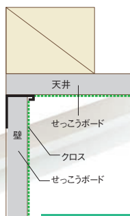
天井勝ち 納まり例
