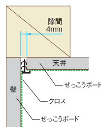
クロス先貼り施工
