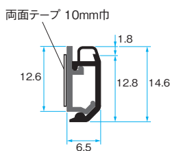
クロス押さえ見切 14
