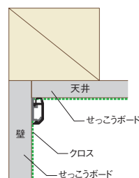
壁勝ち 納まり例
