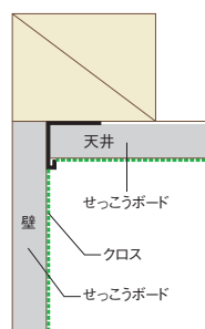
壁勝ち 納まり例
