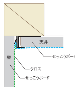
壁勝ち 納まり例
