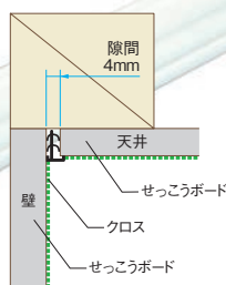
クロス後貼り施工
