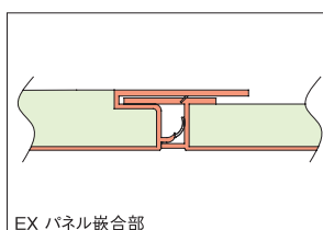
EX パネル嵌合部
