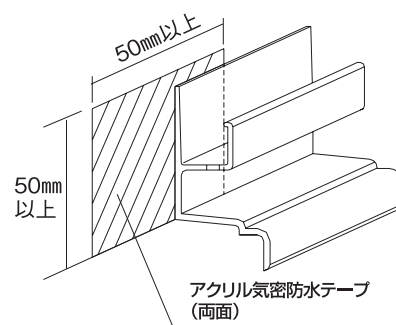
長手のジョイント 突付け+アクリル気密防水テープ裏貼り
