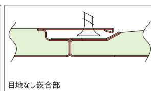
目地なし嵌合部
