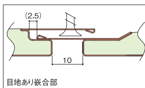
目地あり嵌合部
