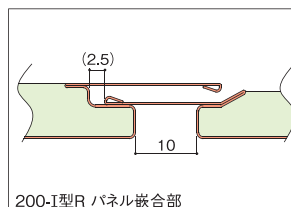
200-I型R パネル嵌合部
