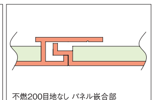
不燃200目地なし パネル嵌合部
