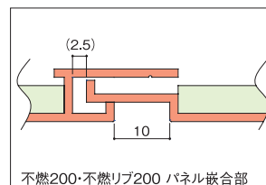
不燃200・不燃リップ200 パネル嵌合部
