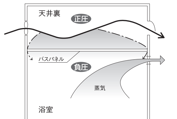
物件(軽量鉄骨下地)施工の天井裏換気方法 第2種機械換気(給気口+排気口)
