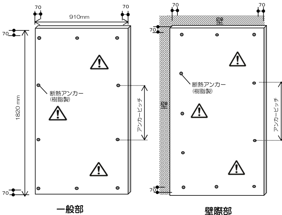
断熱アンカーの端部からの距離
