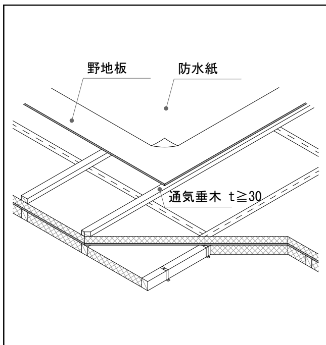
⑤通気垂木施工～⑥野地板・防水紙施工
