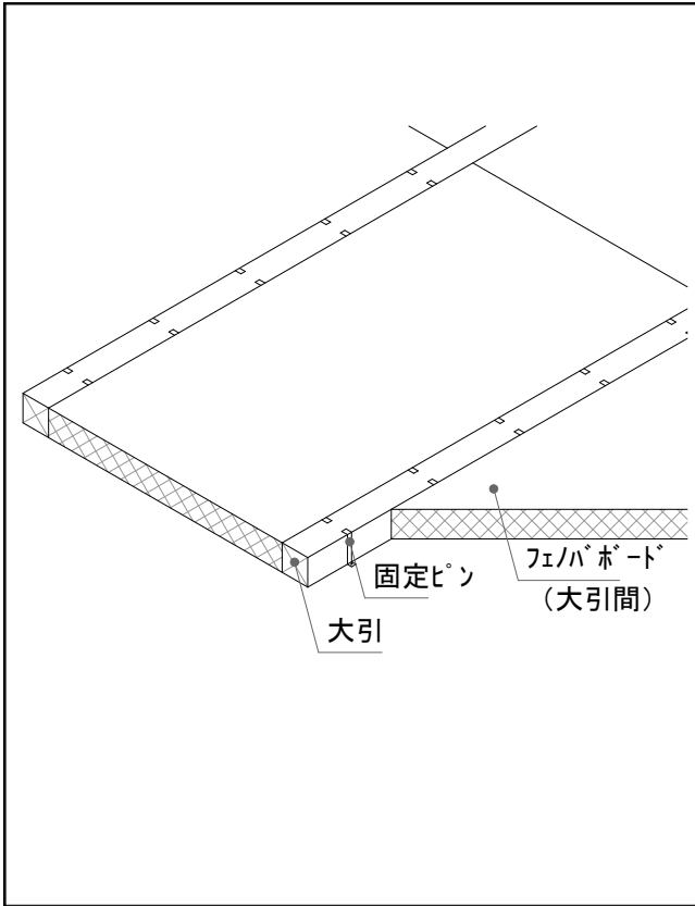
①固定ピン固定～②フェノバボード大引間充填
