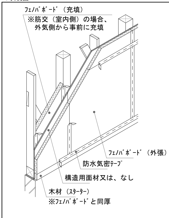
① 構造用面材施工～③ フェノバボード外張
