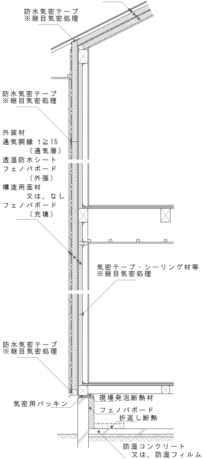
屋根・基礎断熱
