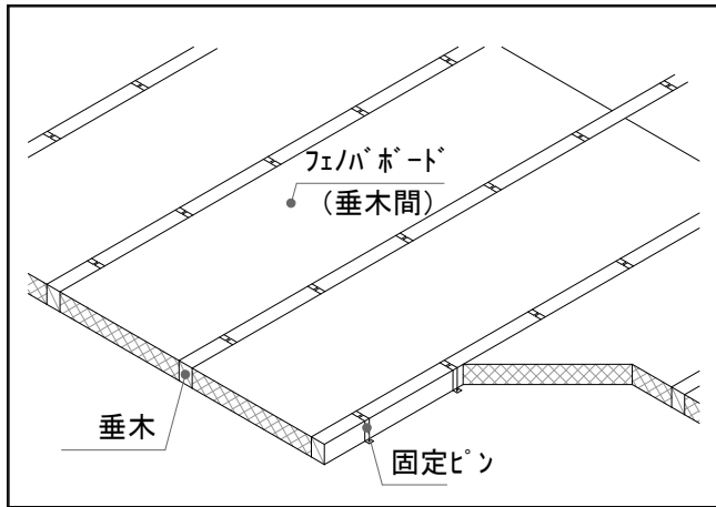
①固定ピン設置～②フェノバボード垂木間充填
