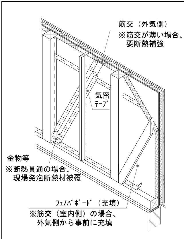
⑦フェノバボード充填
