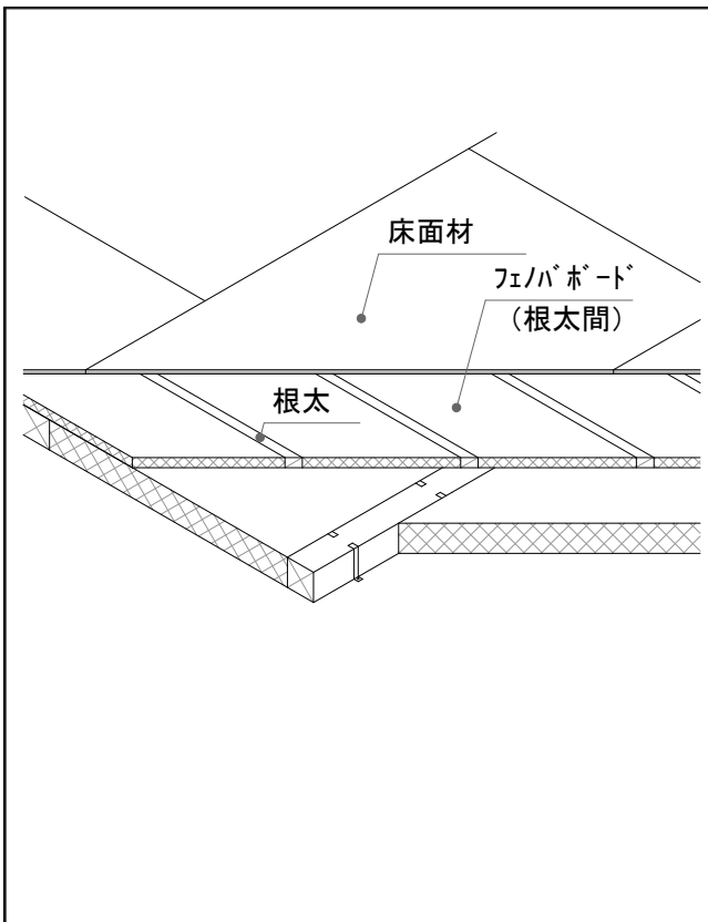
③根太施工～⑤床面材施工
