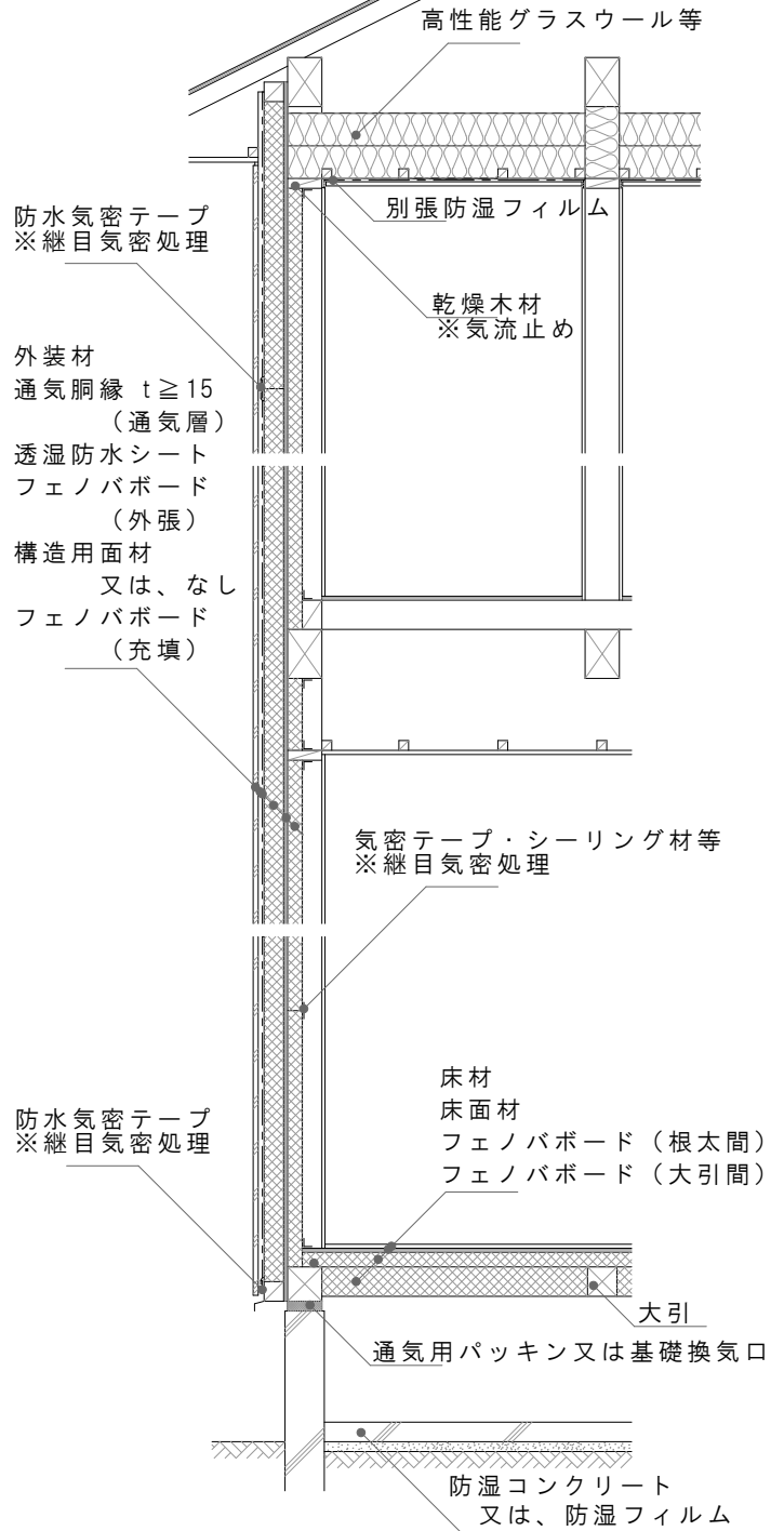
天井・床断熱
