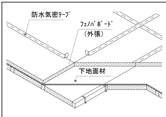
③下地面材施工～④フェノバボード施工
