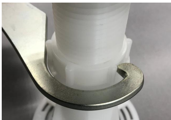
ストッパーに治具の先端を引っ掛けた状態
