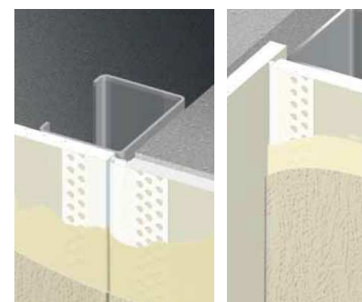
●振動吸收入隅目地CT3
