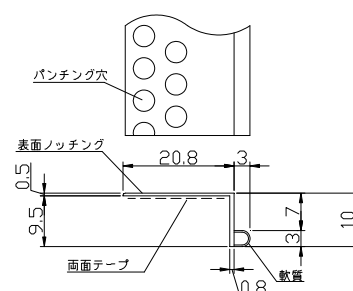
●振動吸收入隅目地CT3
