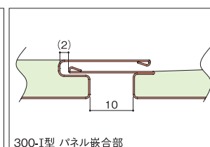
300-I型 パネル嵌合部
