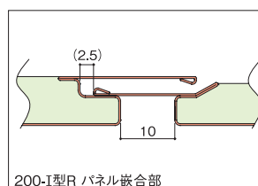
200-I型R パネル嵌合部
