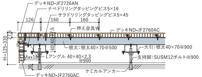
B-B断面図
