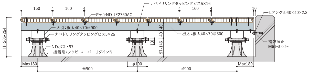
B-B断面図
