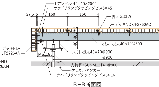
B-B断面図
