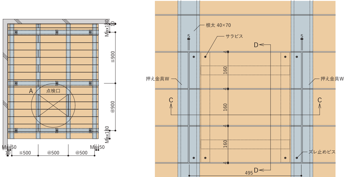
A部詳細
