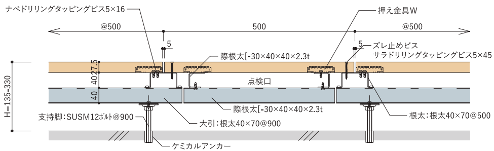
C-C断面図
