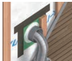
エアコン配管用 (φ75用)
