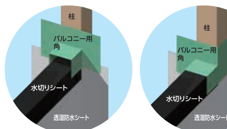
一体タイプ-角
