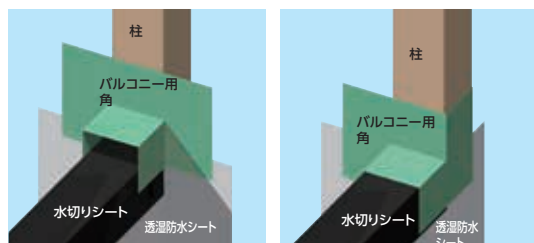
一体タイプ・出入隅
