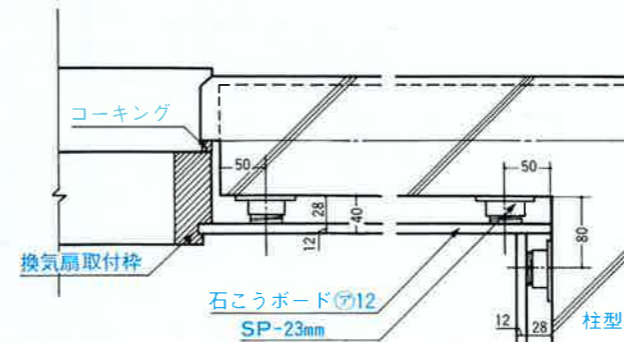
平面詳細図
