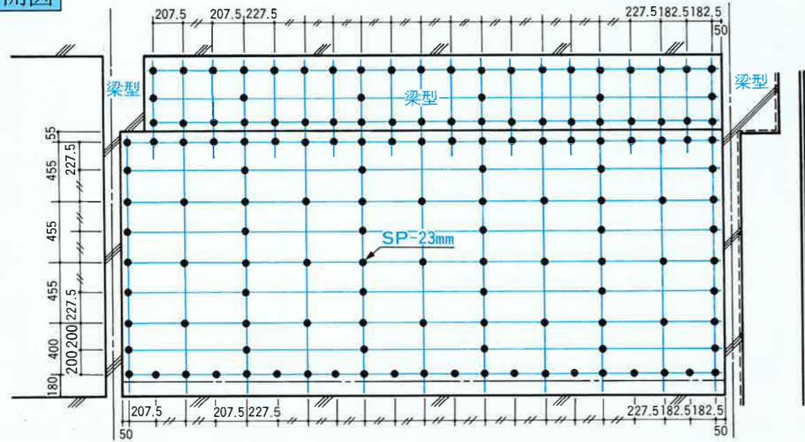
平面図
