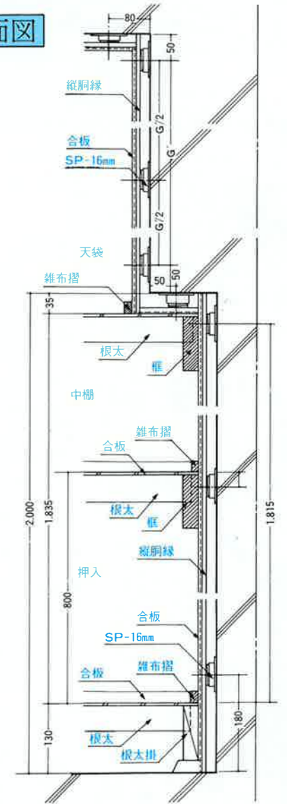
6-6 断面図
