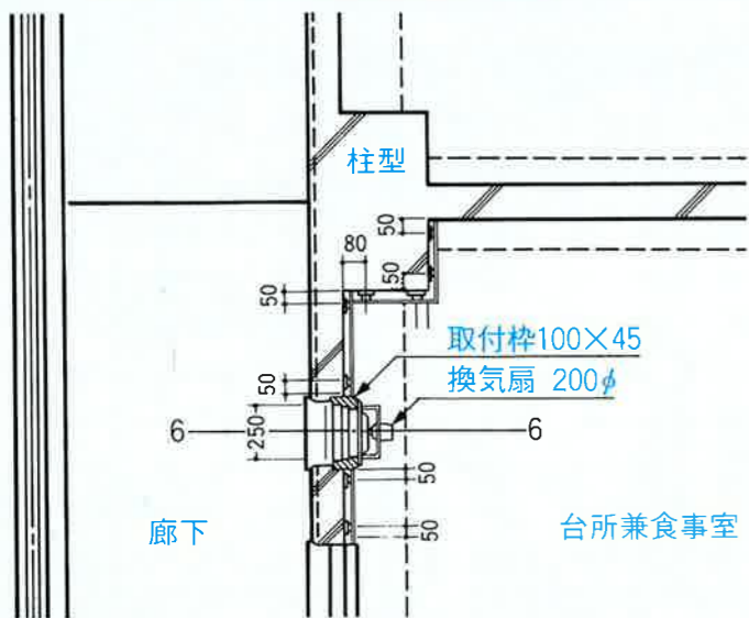
平面図
