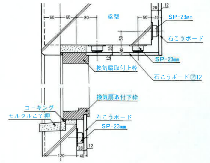
6-6 断面図
