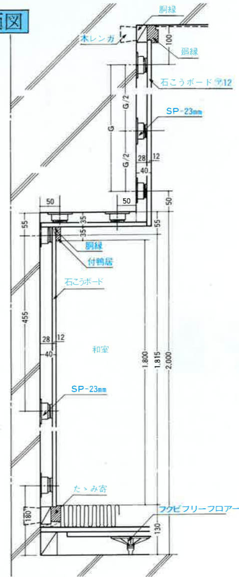
5-5 断面図
