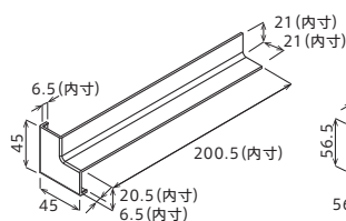
入隅カバー 製品図
