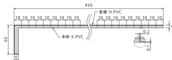
マルチユース窓枠カバー450 製品図
