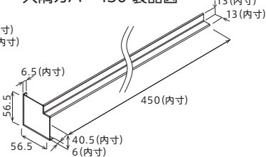
入隅カバー450 製品図
