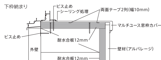
マルチユース窓枠カバー 参考納まり図
