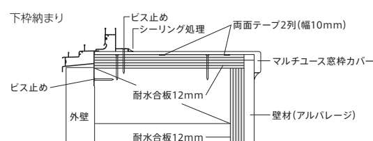
マルチユース窓枠カバー 参考納まり図
