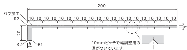
マルチユース窓枠カバー 製品図
