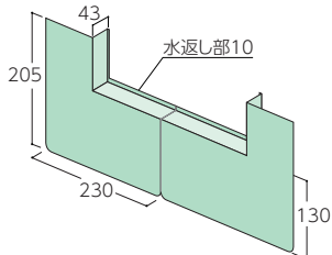
角部材43
