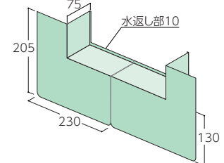
角部材75
