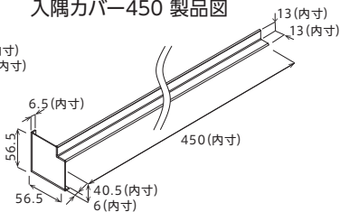
入隅カバー450 製品図
