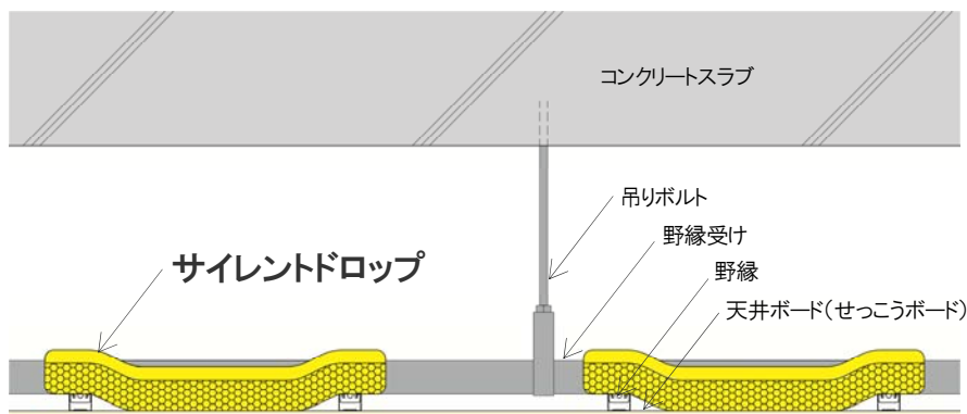
天井断面詳細図
